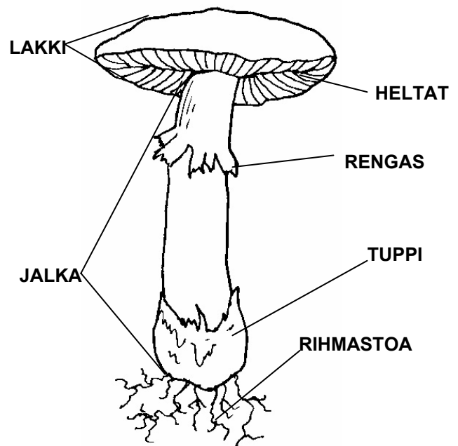
Helttasienen rakenne
